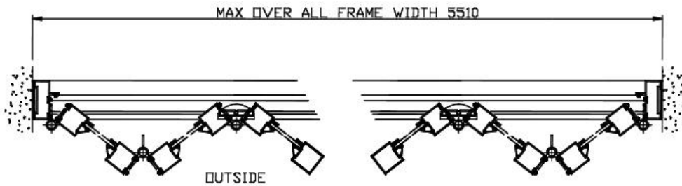
6 PANEL DOOR CONFIGURATION
