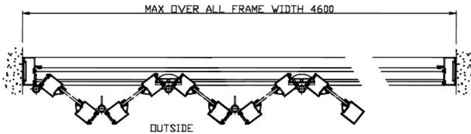
5 PANEL DOOR CONFIGURATION
