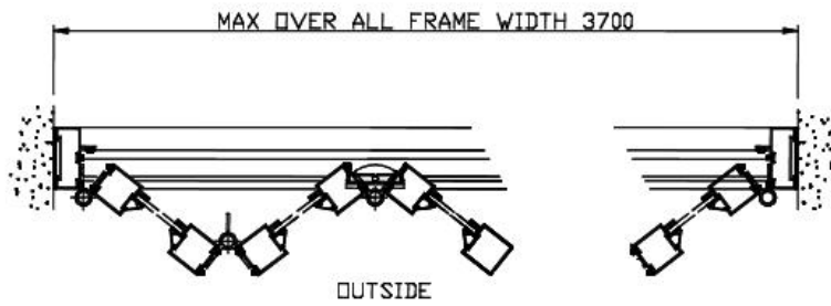
4 PANEL DOOR CONFIGURATION
